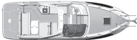
HAUPTDECK
